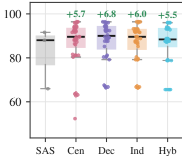
MedQA (USMLE)
