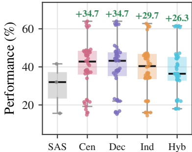
MedXpertQA
