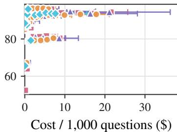
MedQA (USMLE)
