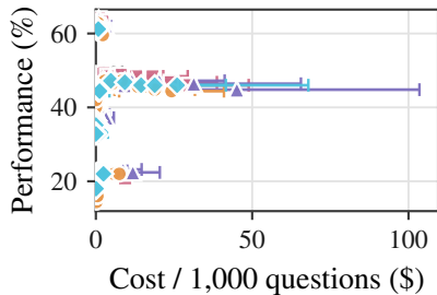
MedXpertQA
