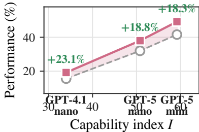
MedXpertQA
