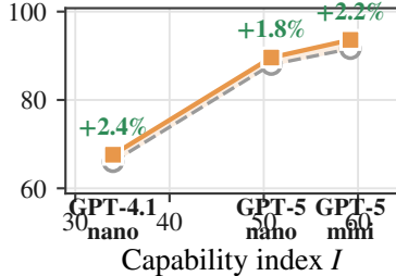
MedQA (USMLE)
