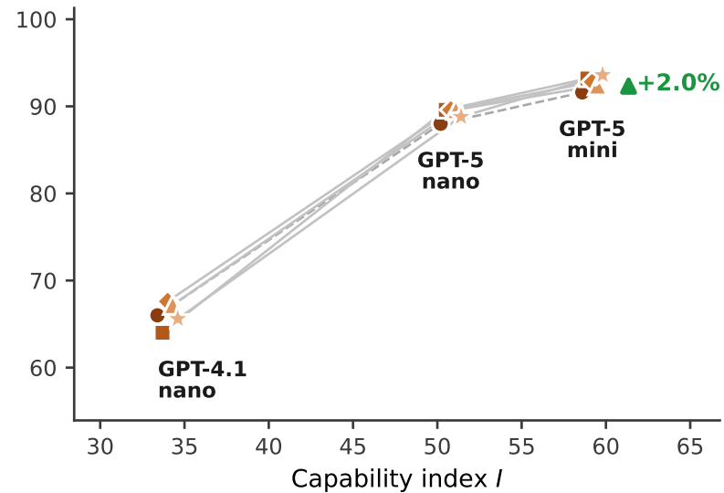
OpenAI GPT · MedQA (USMLE)
