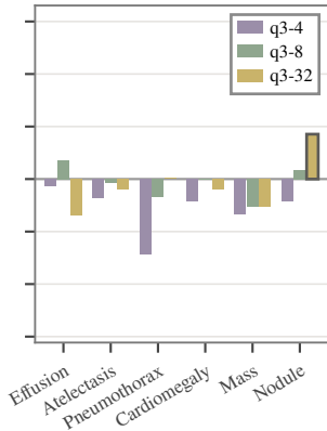
(b) Qwen3-VL on NIH
