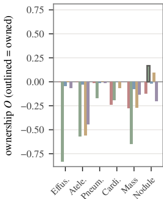
(d) size ladders on NIH
