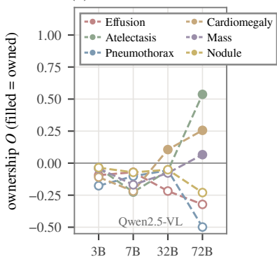
(d) size ladders on NIH
