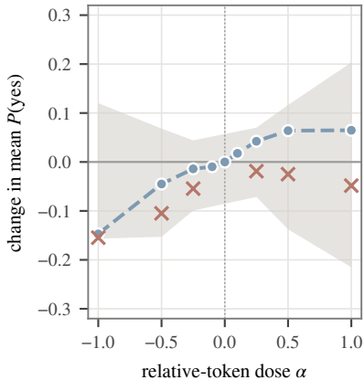
(a) LLaVA-1.5-7B, Effusion
