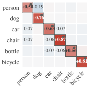
(d) Qwen2.5-VL-7B, COCO
