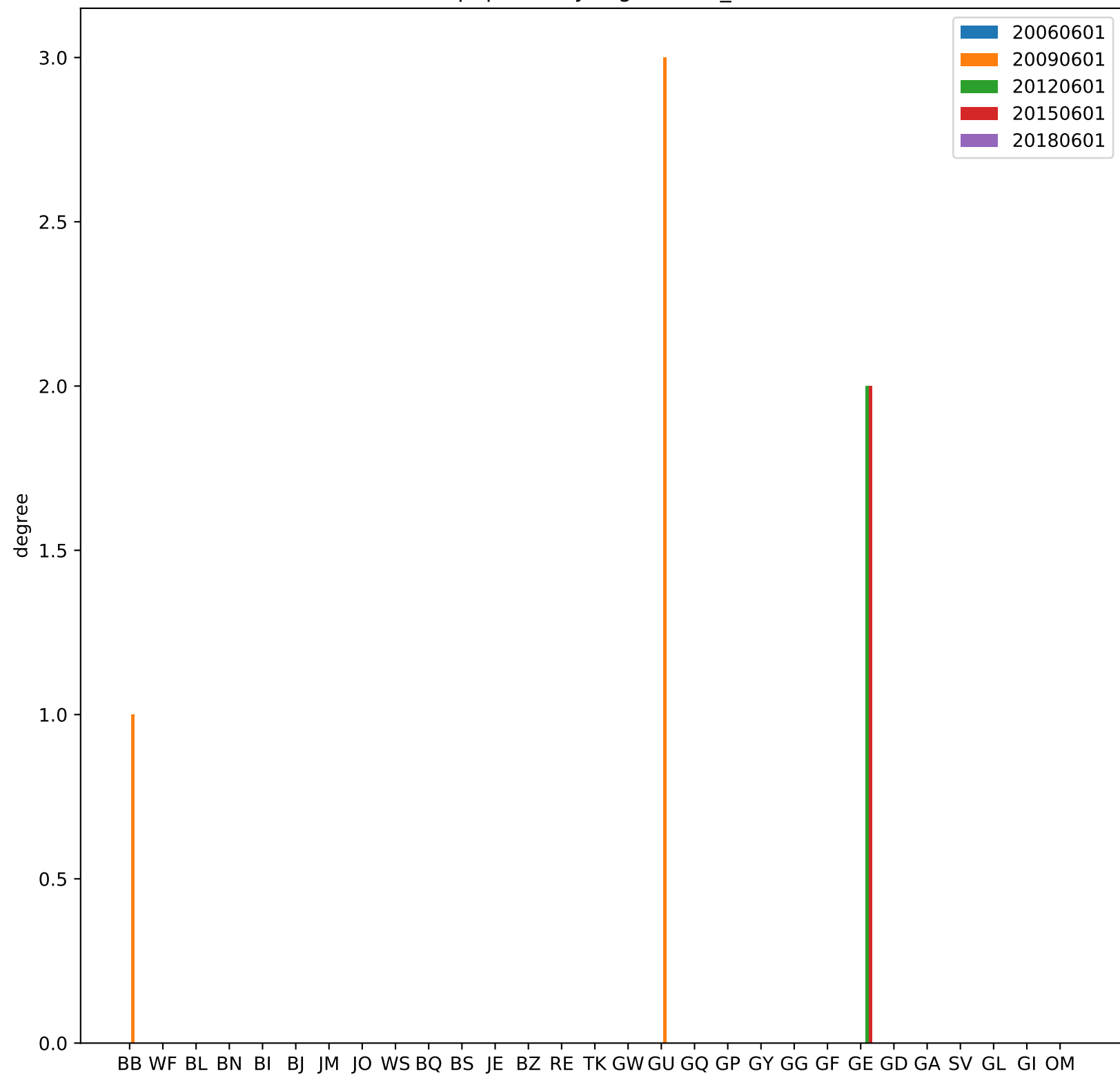
p2pCountryDegreeIntra_0
