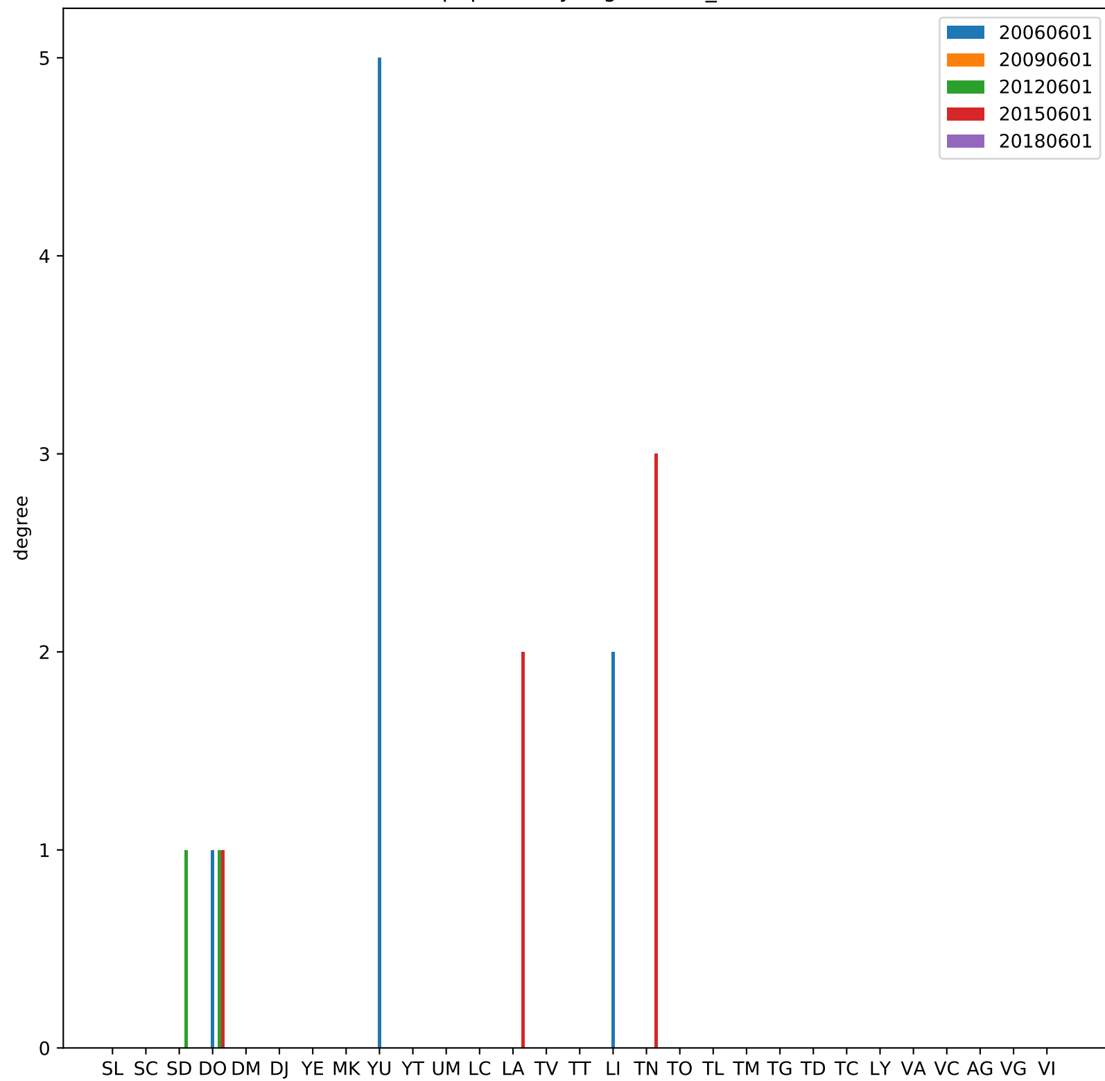
p2pCountryDegreeIntra_3
