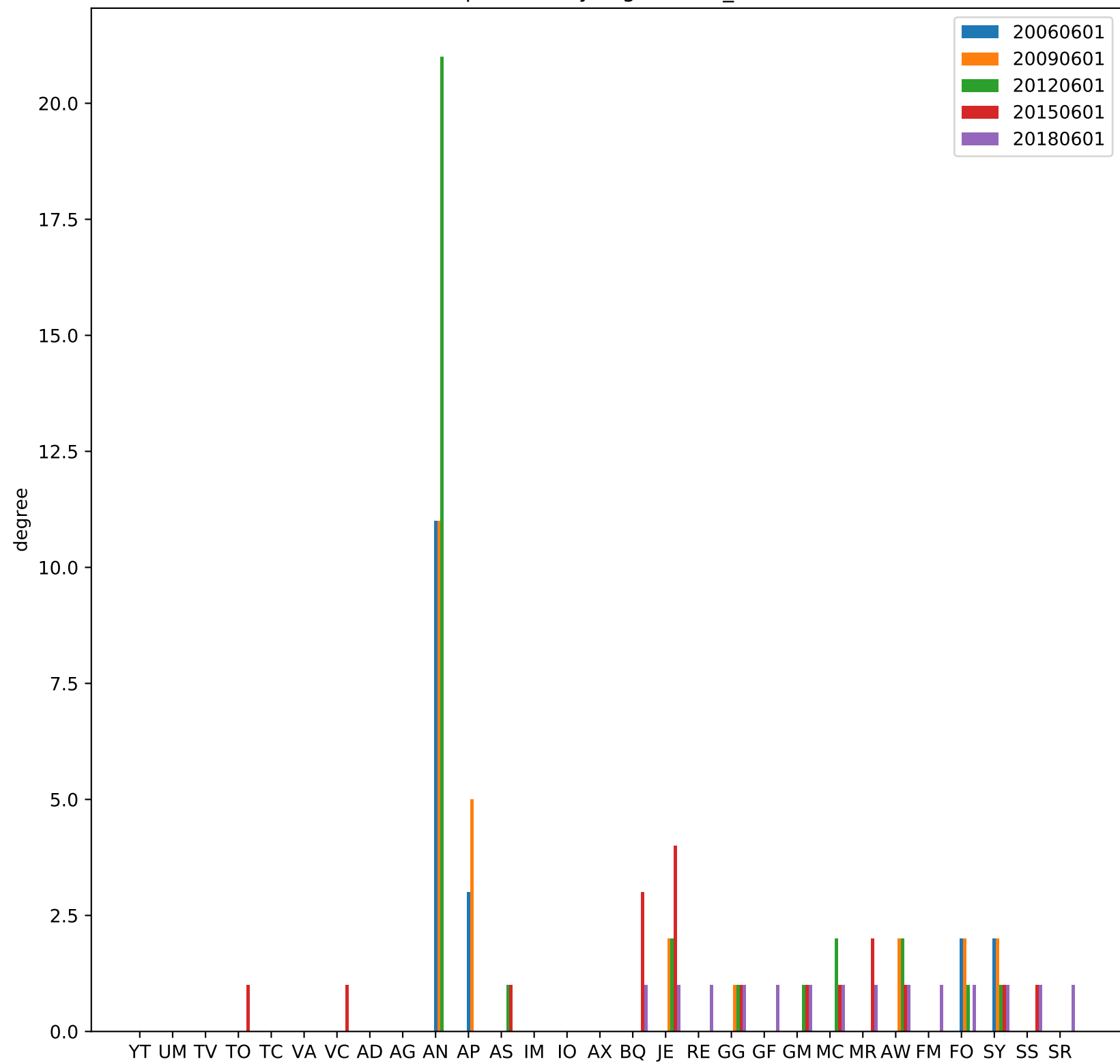
p2cCountryDegreeIntra_1
