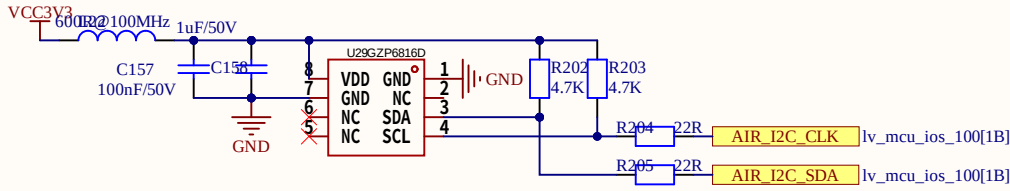
环境气压、温度传感器
