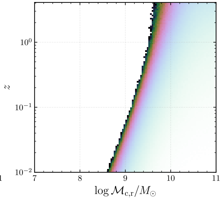
IPTA
