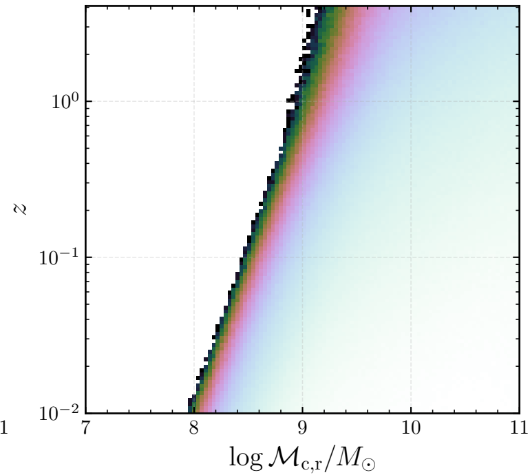
SKA
