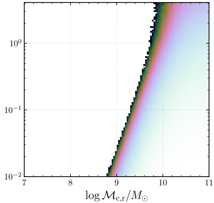
EPTA
