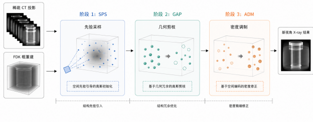
Figure 2: SPAGS 的总体流程。 给定稀疏 CT 投影与 FDK 粗重建, SPS 先把高斯初始化到更有意义的解剖区域, GAP 再回收局部冗余高斯, ADM 最后进行位置相关的密度修正, 从而生成目标新视角 X 射线投影。
