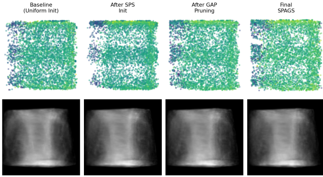
Figure 9: 高斯空间分布的逐步收紧过程。从均匀初始化到 SPS 引导初始化，再到 GAP 剪枝与最终 SPAGS ，高斯支撑逐步贴合有效结构区域，对应投影结果也随之更加稳定。
