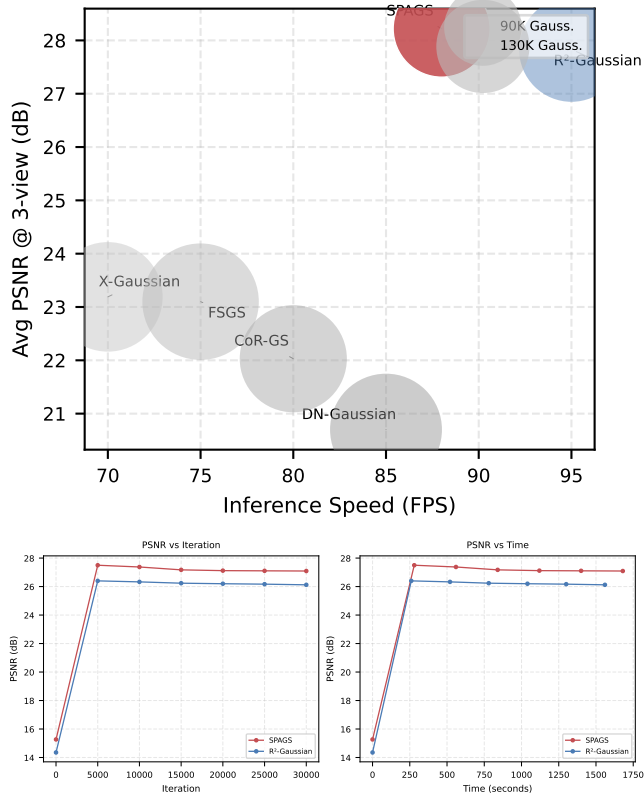
Figure 10: 效率与收敛分析。上: 不同方法的 PSNR-FPS 权衡, 圆点大小表示最终 Gaussian 数量; 下: SPAGS 与 R^2-Gaussian 在 3-view Chest 场景上的 PSNR 收敛曲线, 分别按迭代次数和 wall-clock time 统计, 用于展示额外训练开销与性能收益的关系。
