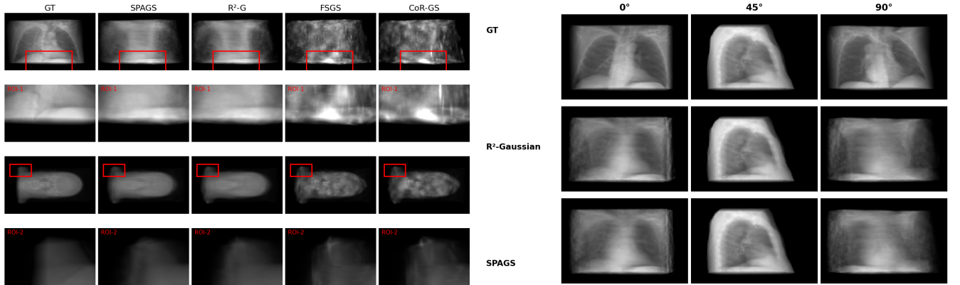
Figure 7: 局部细节与跨视角一致性分析。左：两组放大 ROI，对比肋骨/颅骨边界附近的局部结构与软组织过渡。右：同一病例在三个目标角度下的结果，SPAGS 相比 R^2 -Gaussian 保持了更稳定的跨视角形态，并减少了角度特异性伪影。
