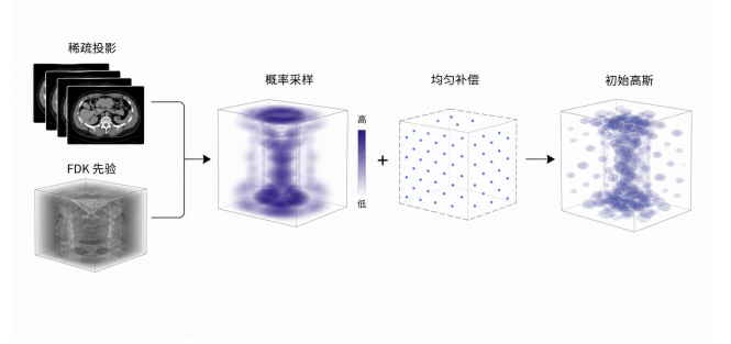
Figure 3: SPS 模块示意。 利用 FDK 粗重建引导密度加权采样, 使更多初始高斯落在解剖相关区域, 同时保留少量均匀补偿采样以维持全局覆盖。
