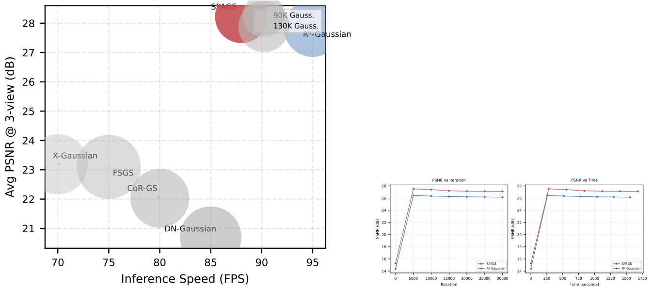
Figure 10: 效率与收敛分析。左：不同方法的 PSNR -FPS 权衡，圆点大小表示最终 Gaussian 数量。右：SPAGS 与 R^2 -Gaussian 在 3-view Chest 场景上的 PSNR 收敛曲线，分别按迭代次数和 wall-clock time 统计。
