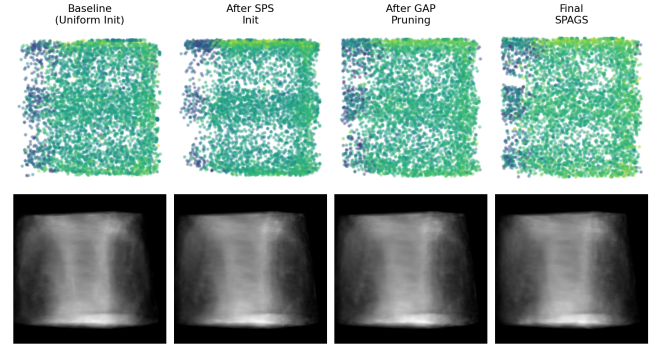
Figure 9: 高斯空间分布的逐步收紧过程。从均匀初始化到 SPS 引导初始化，再到 GAP 剪枝与最终 SPAGS，高斯支撑逐步贴合有效结构区域。
