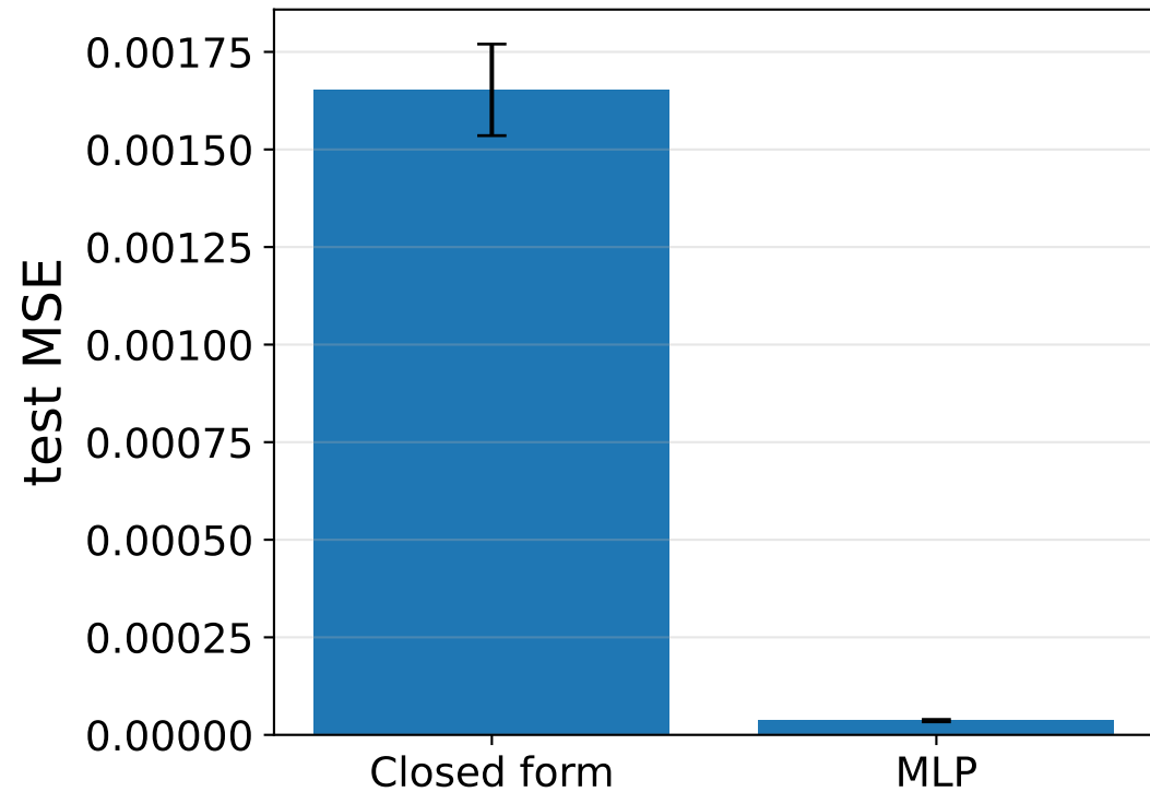
Test error
