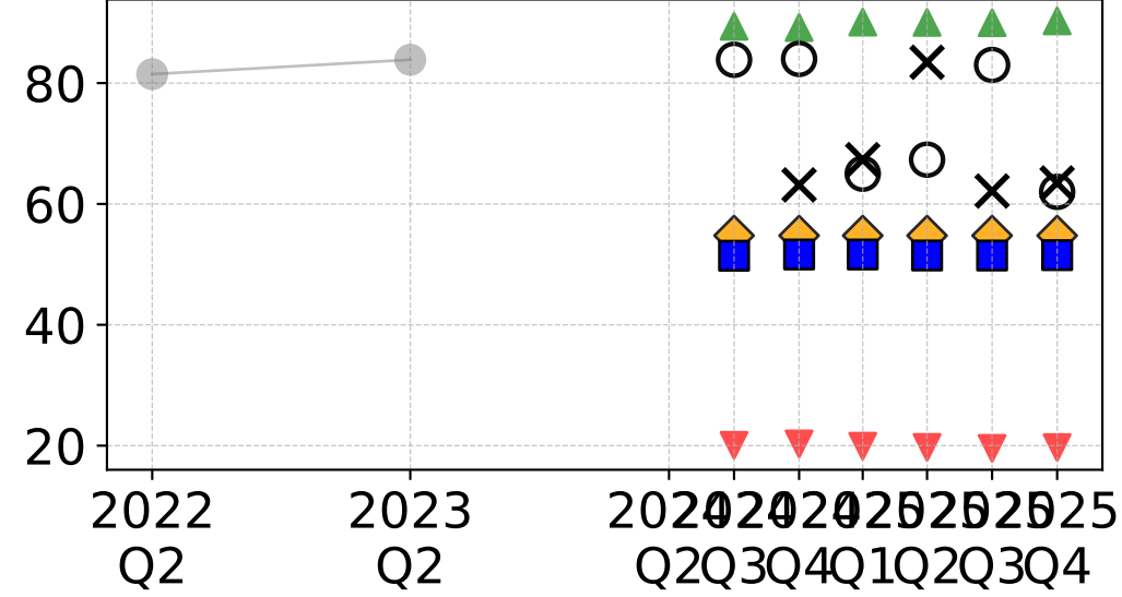
theta_DPO
