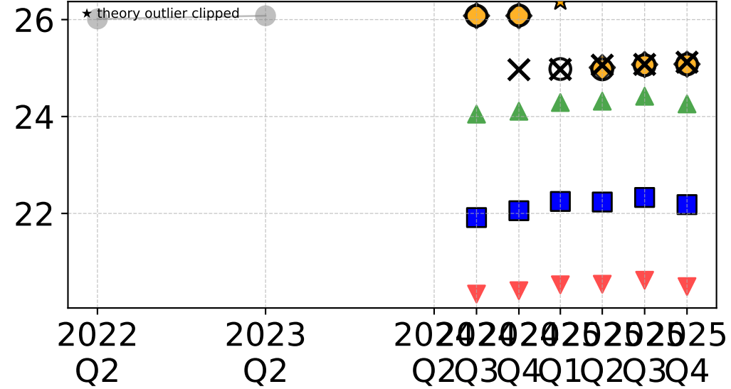
theta_m_opex
