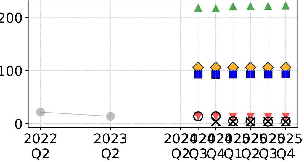
theta_alpha_OCA
