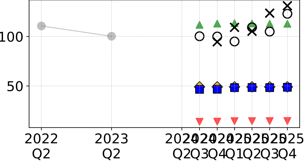
theta_alpha_ONCA
