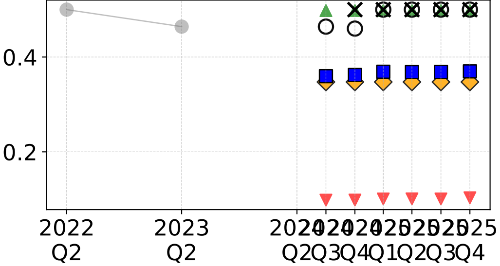
theta_alpha_OCL
