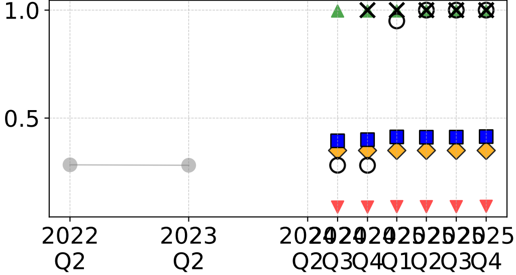
theta_alpha_ONCL
