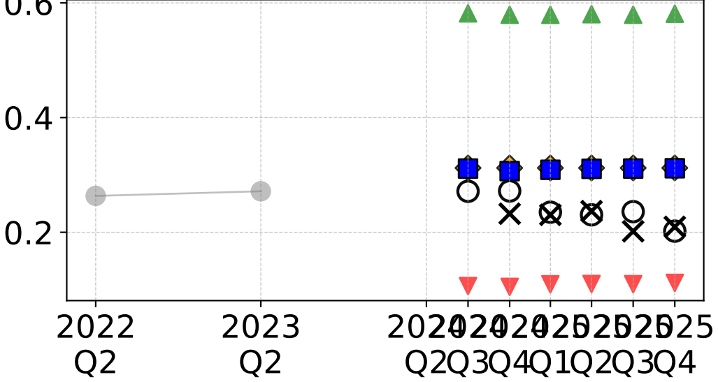
theta_DIO
