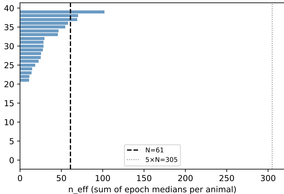
Roaming n_{\text{eff}} per animal ( \tau=20.0\text{s} , W=10.0\text{s} , MB=10.0\text{s} )
