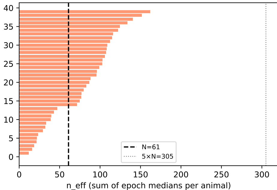
Non-roaming n_{\text{eff}} per animal ( \tau=20.0\text{s} , W=10.0\text{s} , MB=10.0\text{s} )
