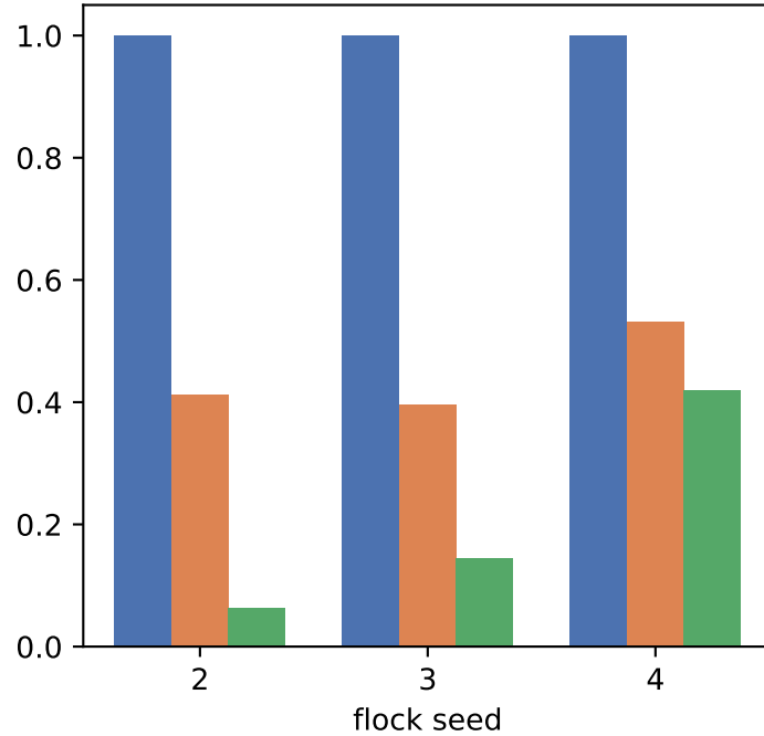
final R_0
