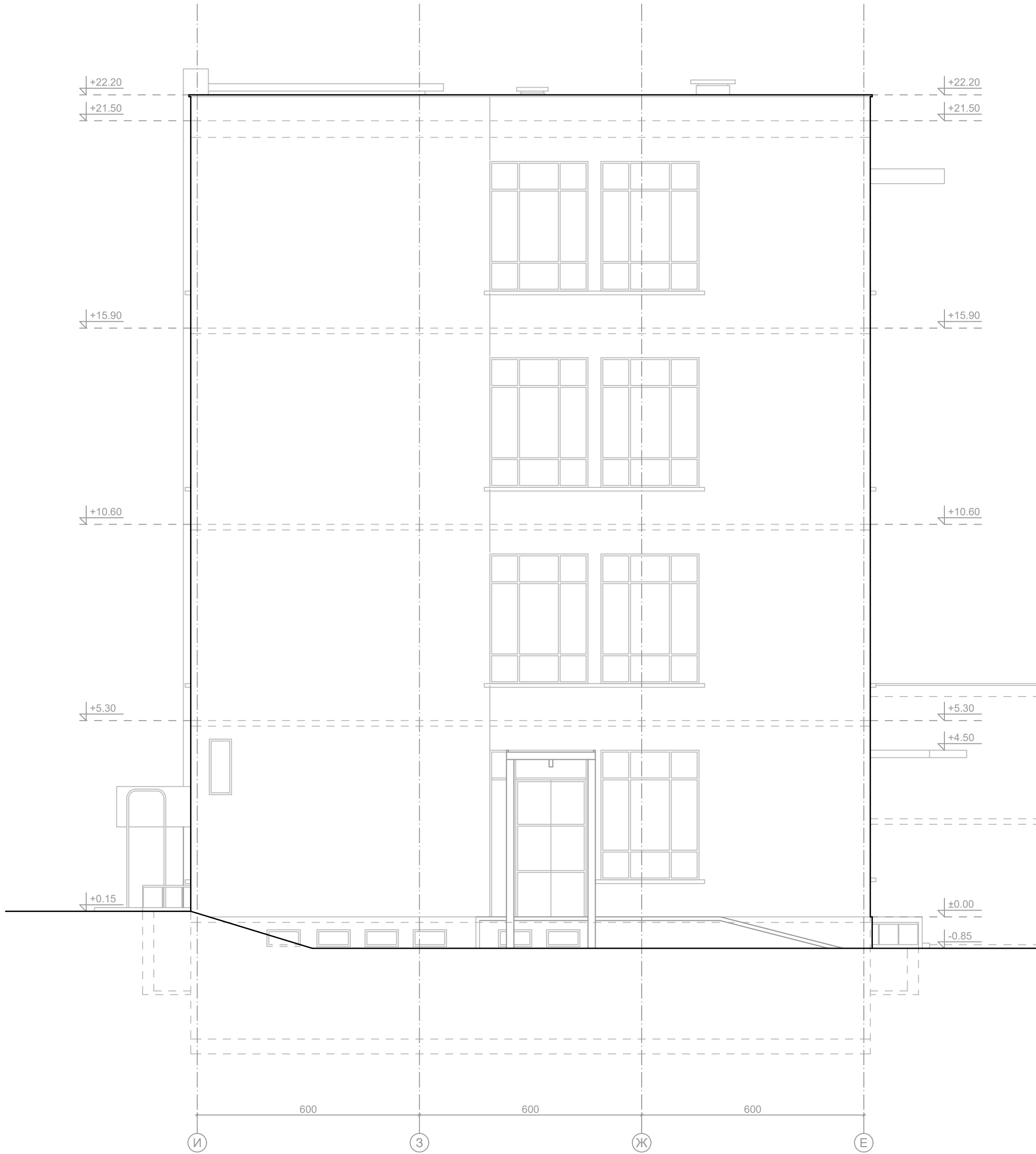
Тяло 1 Фасада ЮГ
