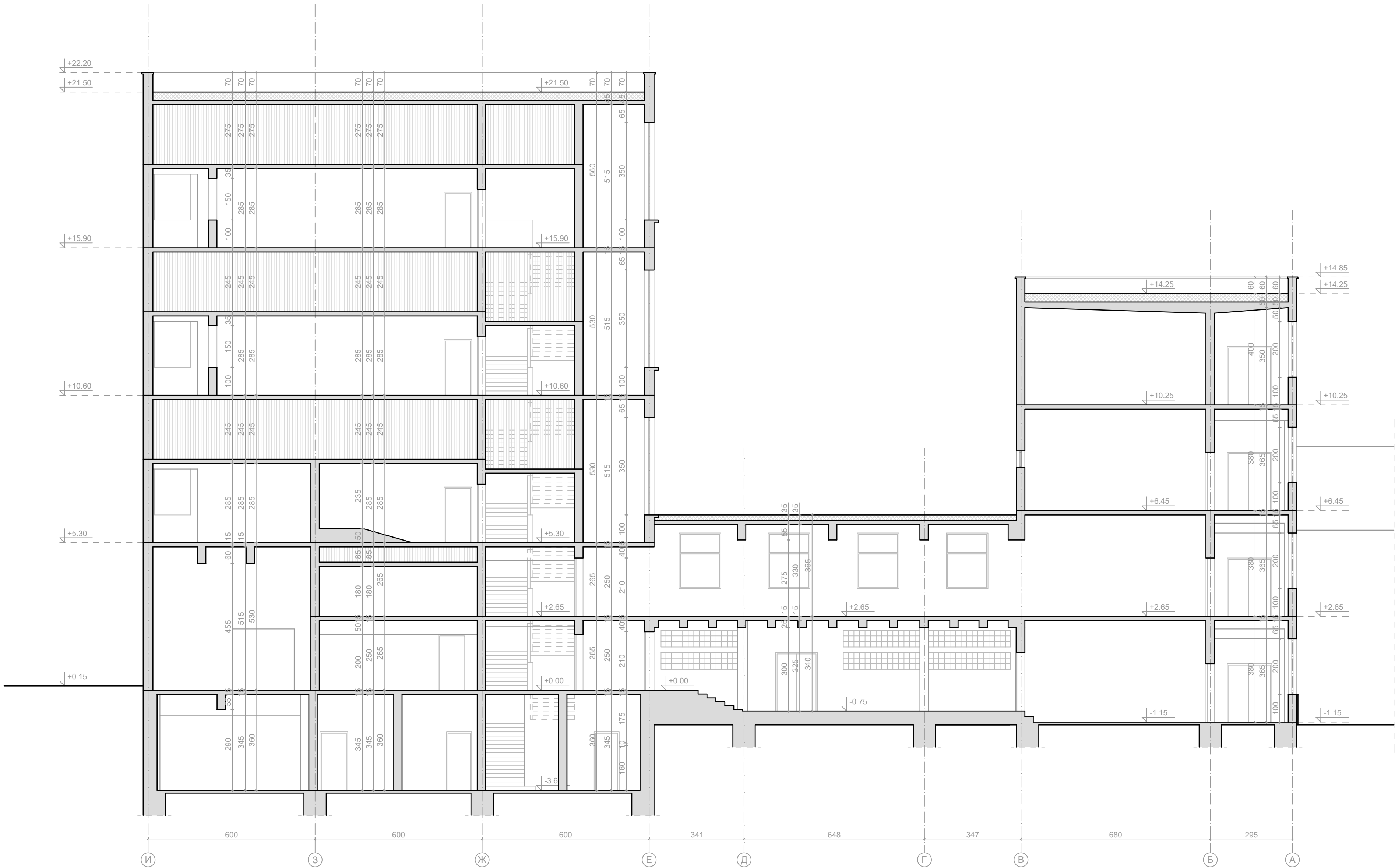
Разрез Б-Б
