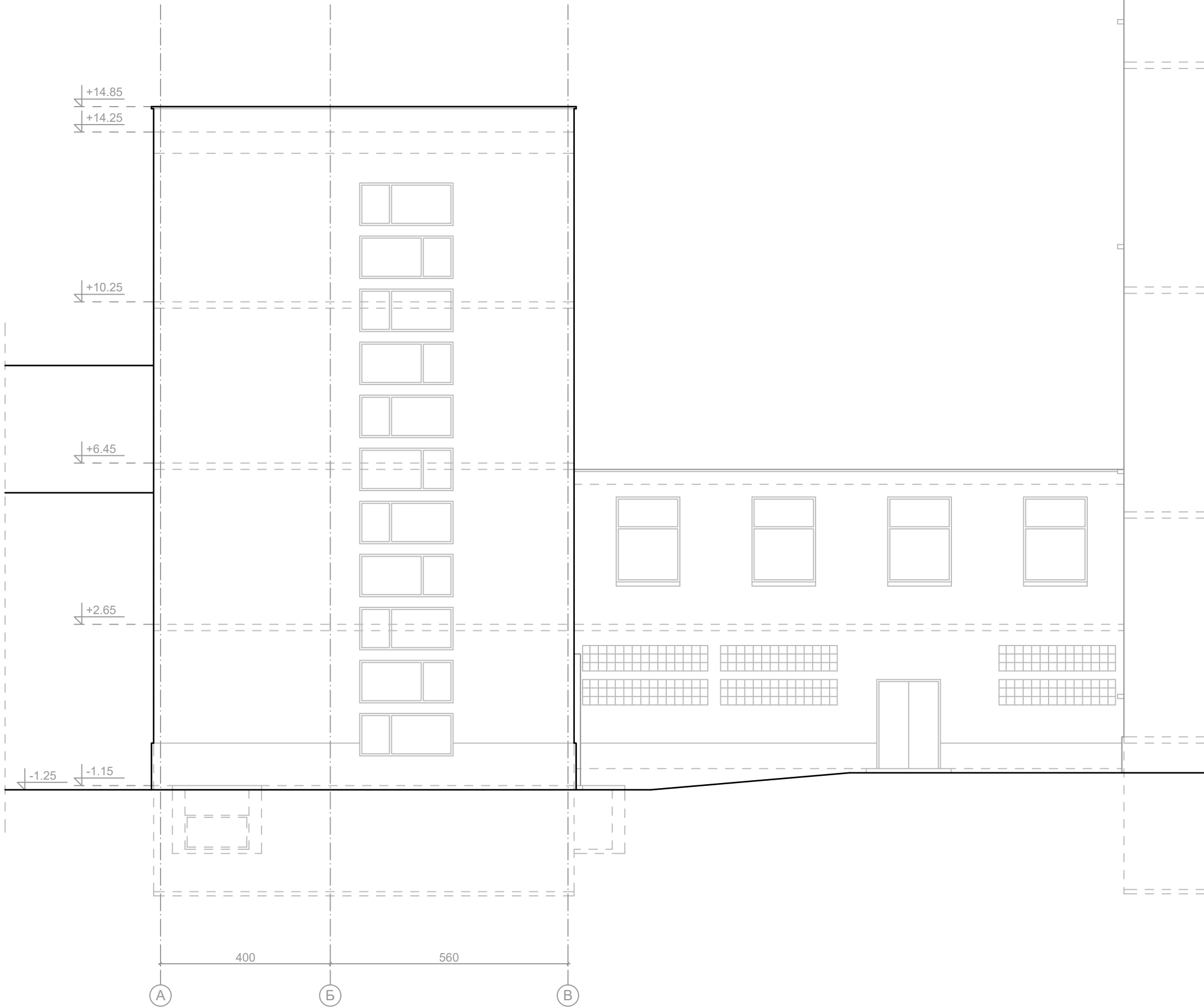
Тяло 2 и топла връзка Фасада СЕВЕР
