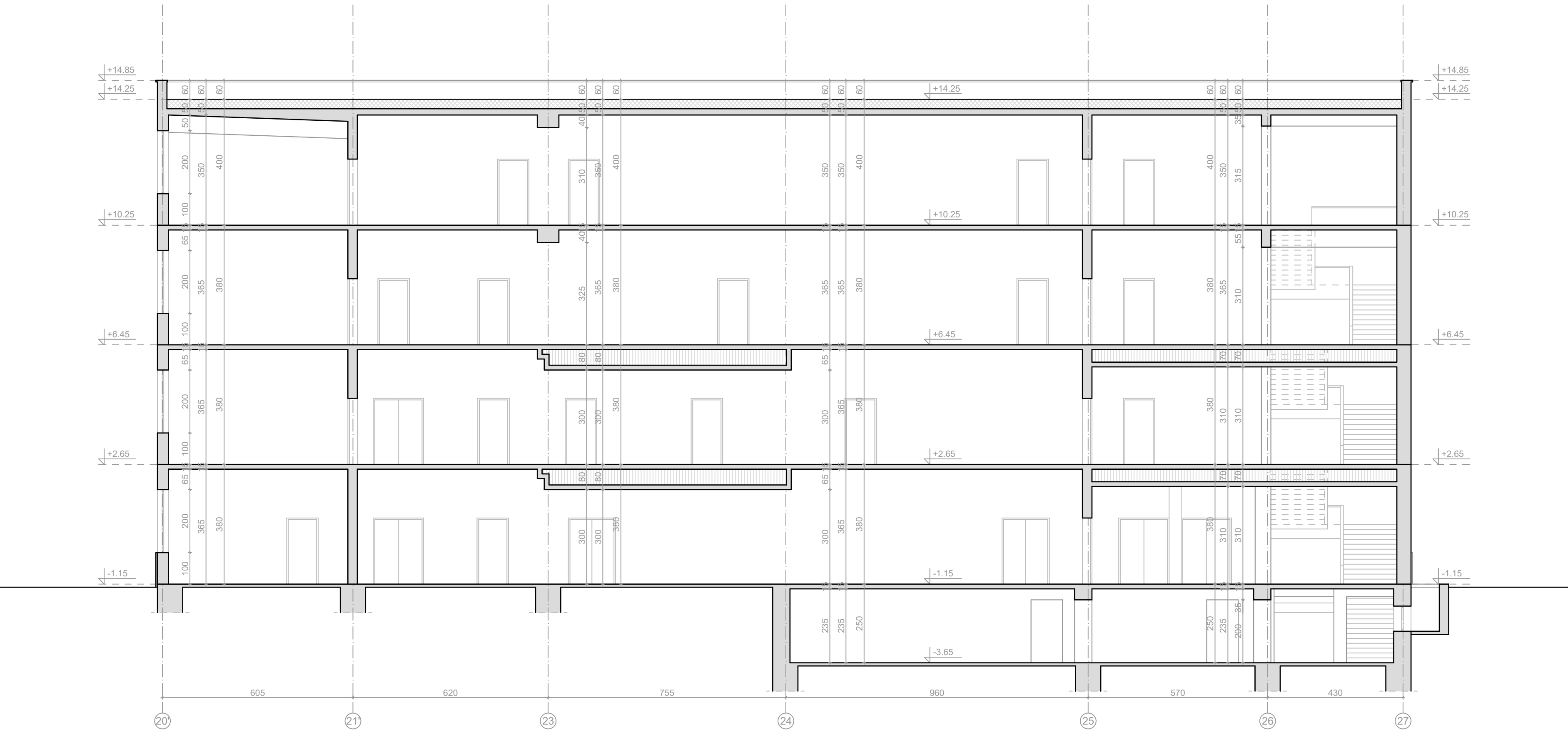
Разрез 2-2
