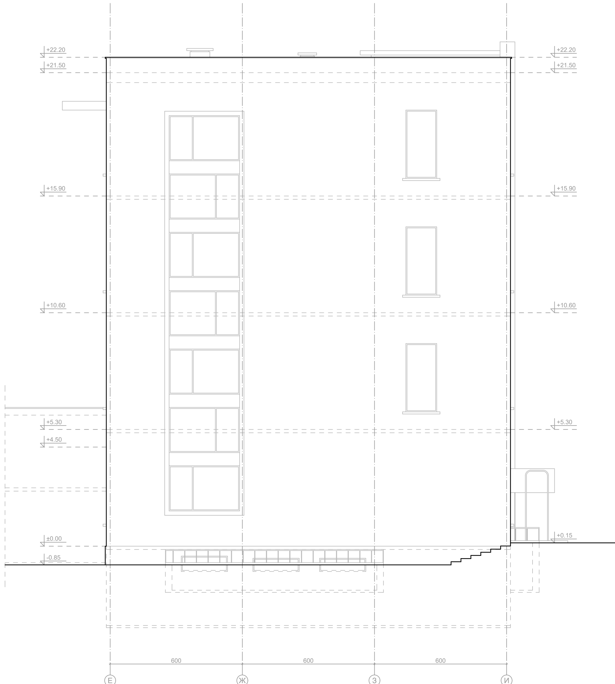
Тяло 1 Фасада СЕВЕР
