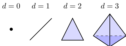
图 14-10: 单纯形
