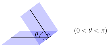
图 11-2: 二面角
