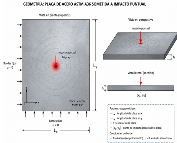
Figura 1: Esquema de la placa bidimensional utilizada en la simulación numérica, indicando la región de impacto central y la propagación dinámica de esfuerzos.
