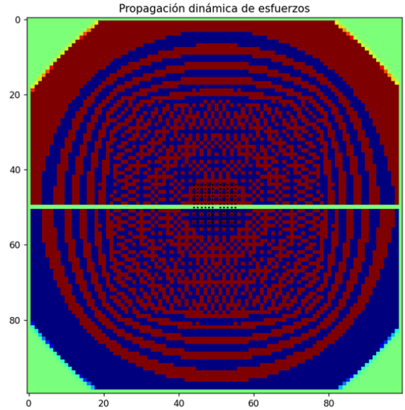
Figura 2: Propagación dinámica de esfuerzos e iniciación localizada de grieta en la placa de acero ASTM A36 sometida a impacto puntual. Las regiones rojas representan esfuerzos de tensión, mientras que las regiones azules representan esfuerzos de compresión.
