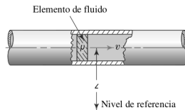
FIGURA 6.4 Elemento de un fluido en una tubería.
