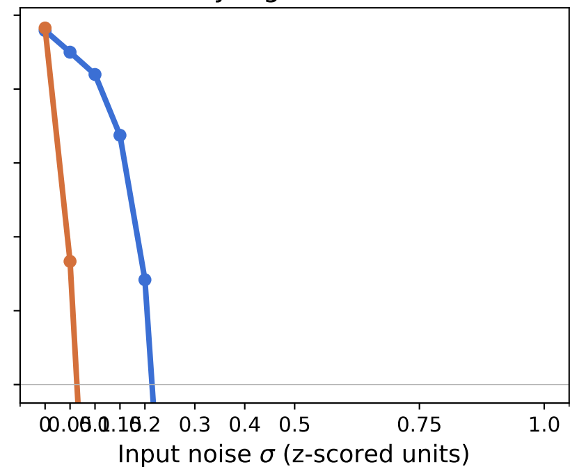
Rayleigh-Bénard
