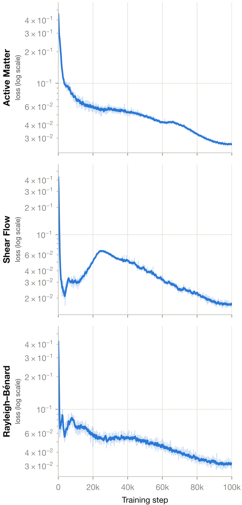
V-JEPA
