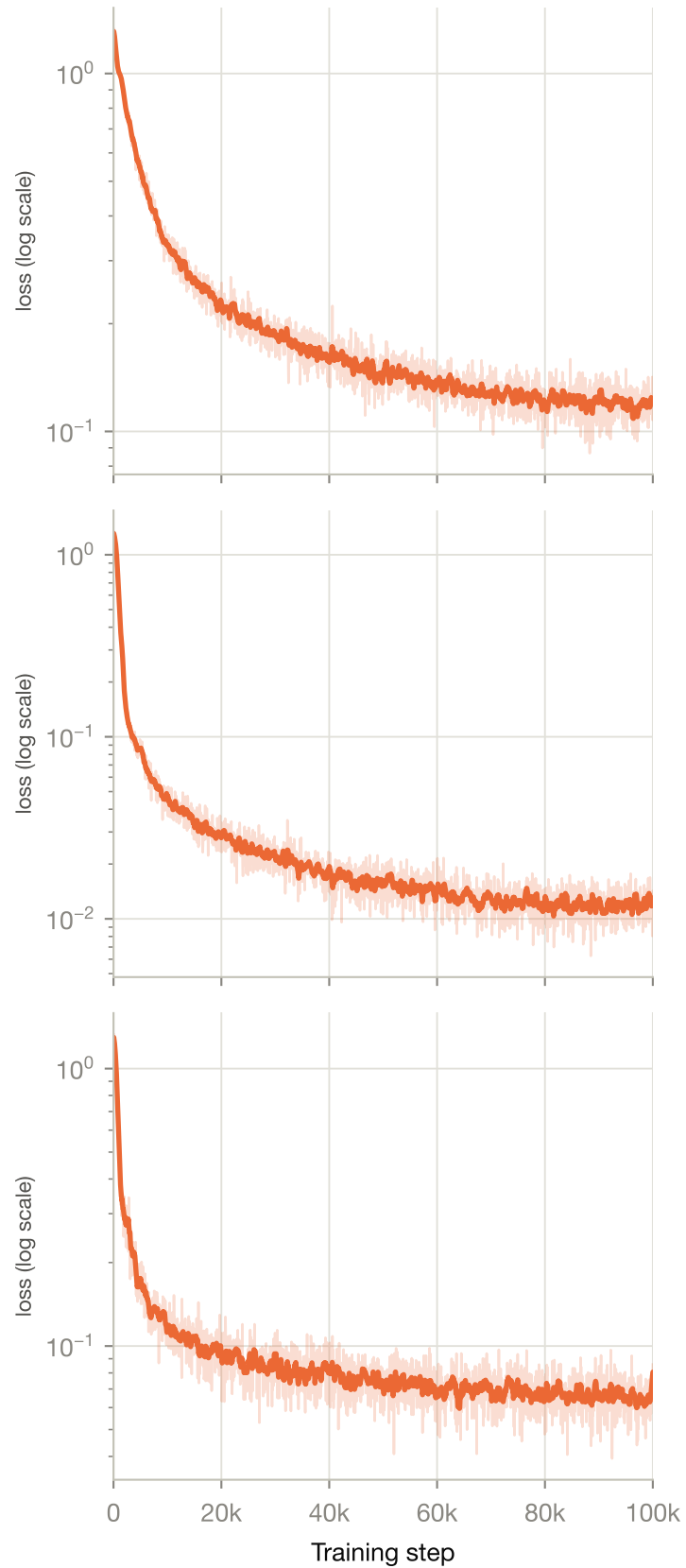
VideoMAE
