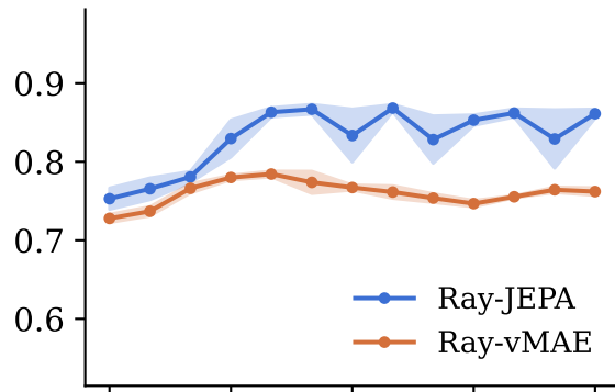
Buoyancy grad.
