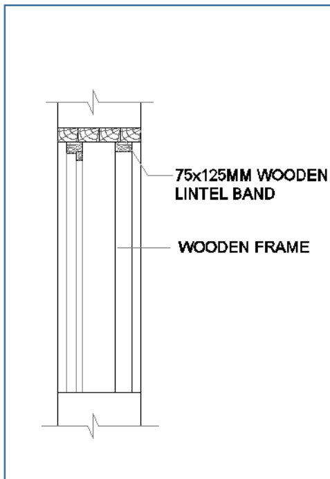
Door Section
