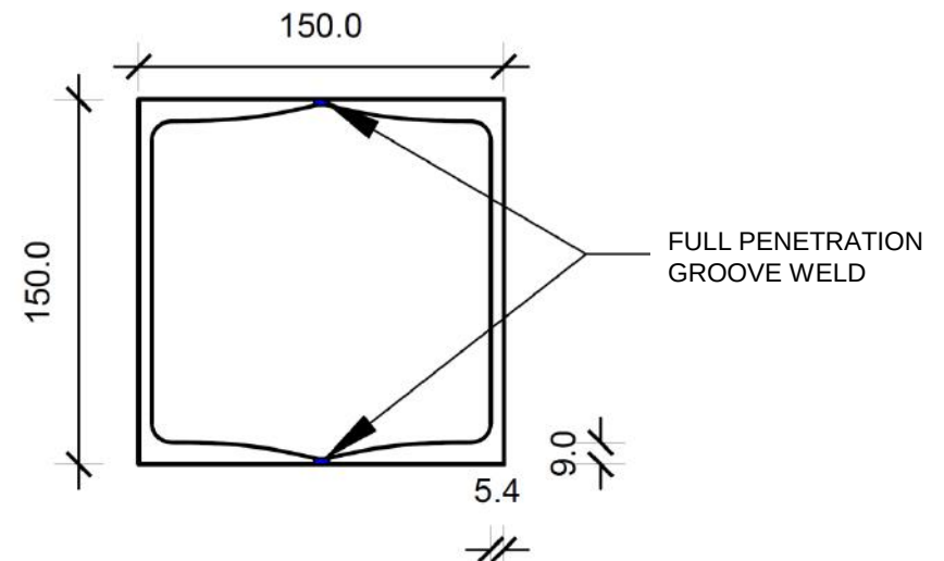
2-ISMC150(COLUMN)
