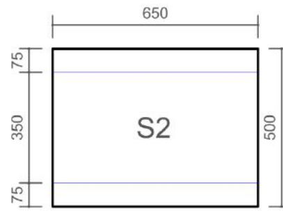
SLAB(S2) DETAILS
