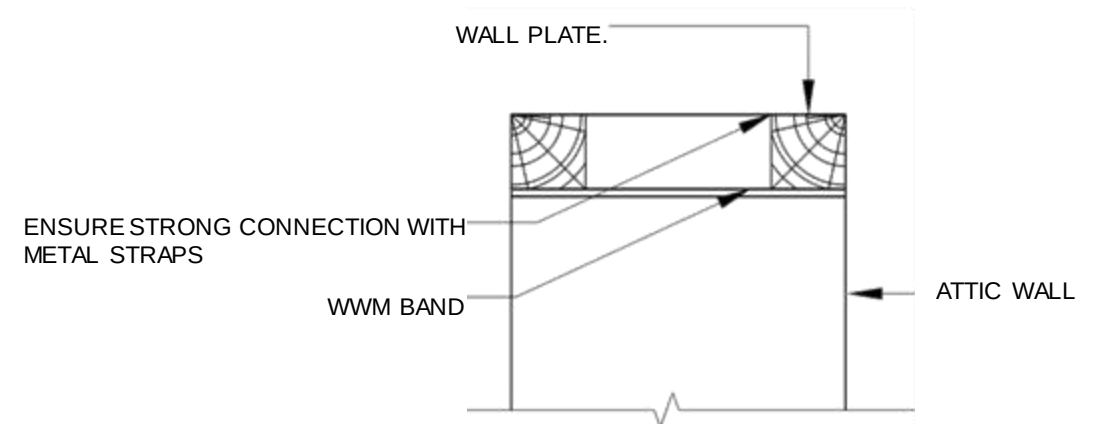
SECTION : D-D
