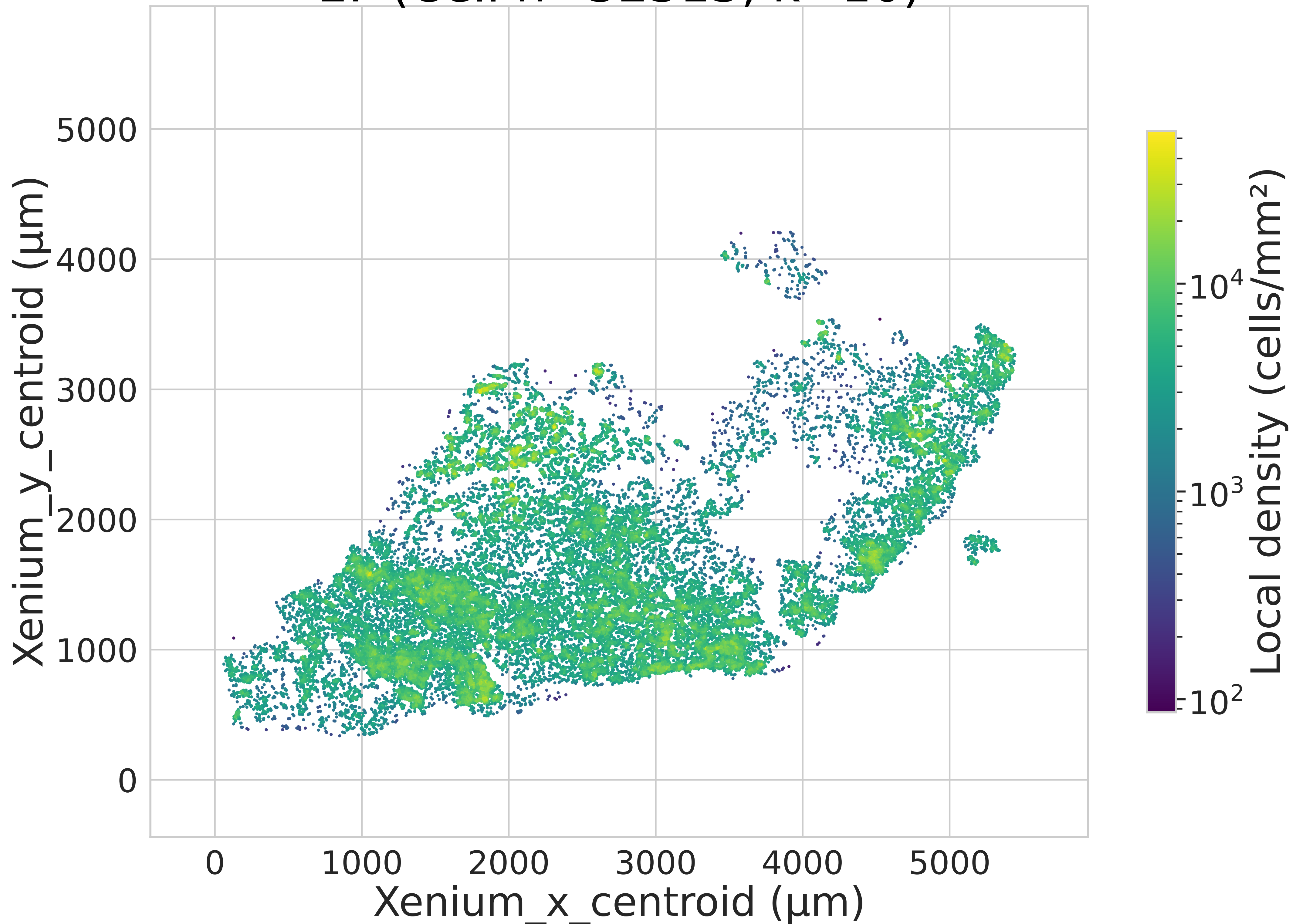
L7 (Cell n=32313, k=10)
