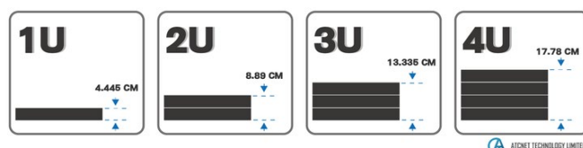
U數:機架式伺服器的高度單位 (1U=4.45cm)
