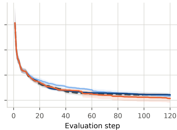
LogEI
