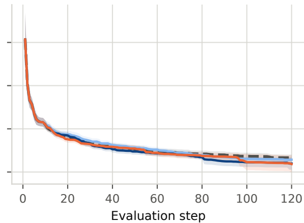
MES-Gumbel
