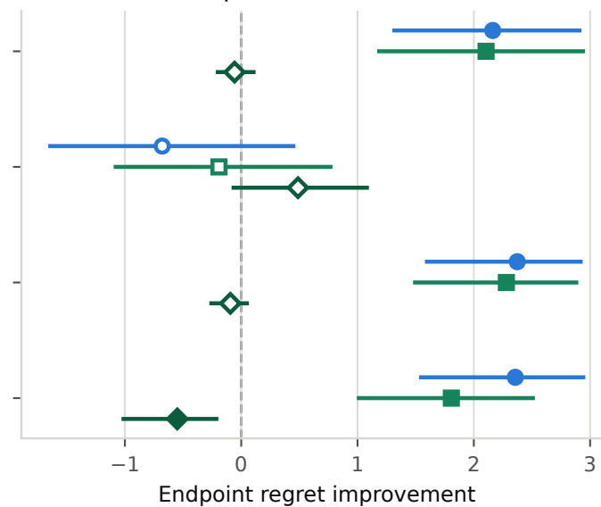
Sparse Hartmann
