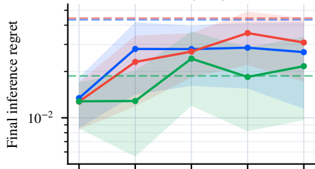
Trid (10D)
