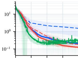
Griewank (10D)
