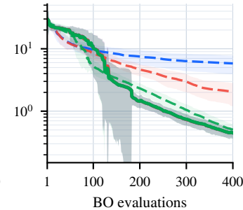
Griewank (30D)
