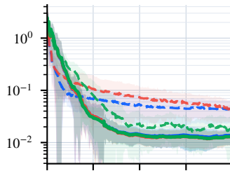
Trid (10D)
