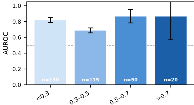
D-MPNN
