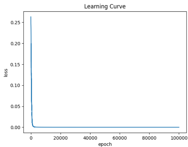
(b) XOR
