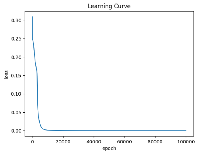
(b) XOR
