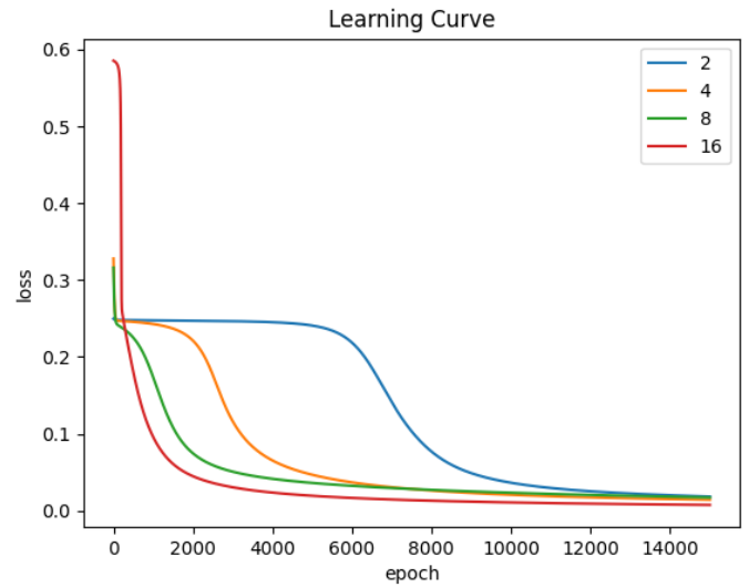
(b) XOR
