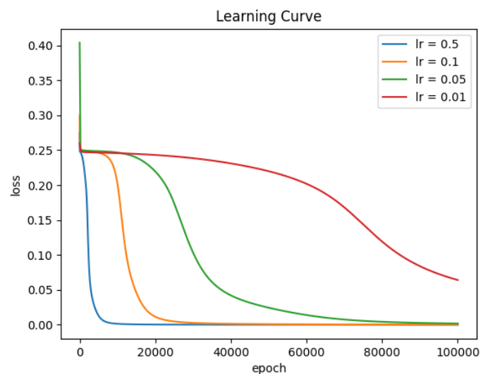
(b) XOR
