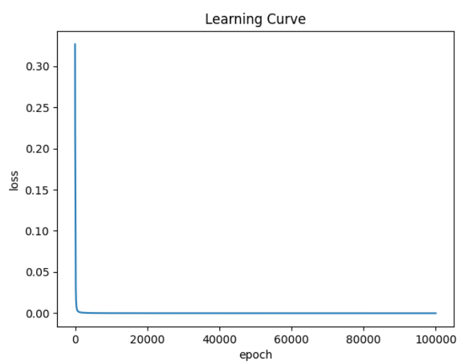
(b) XOR
