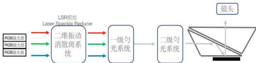
(MALC 目氦三色激光光机架构示意图)
