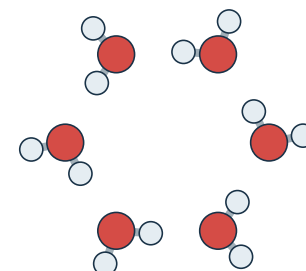
Hexamer
