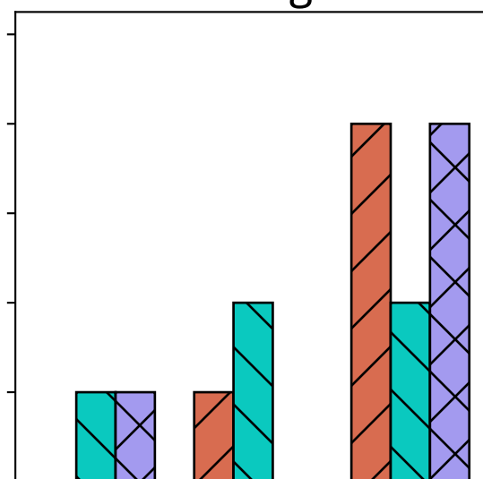
izanagi
