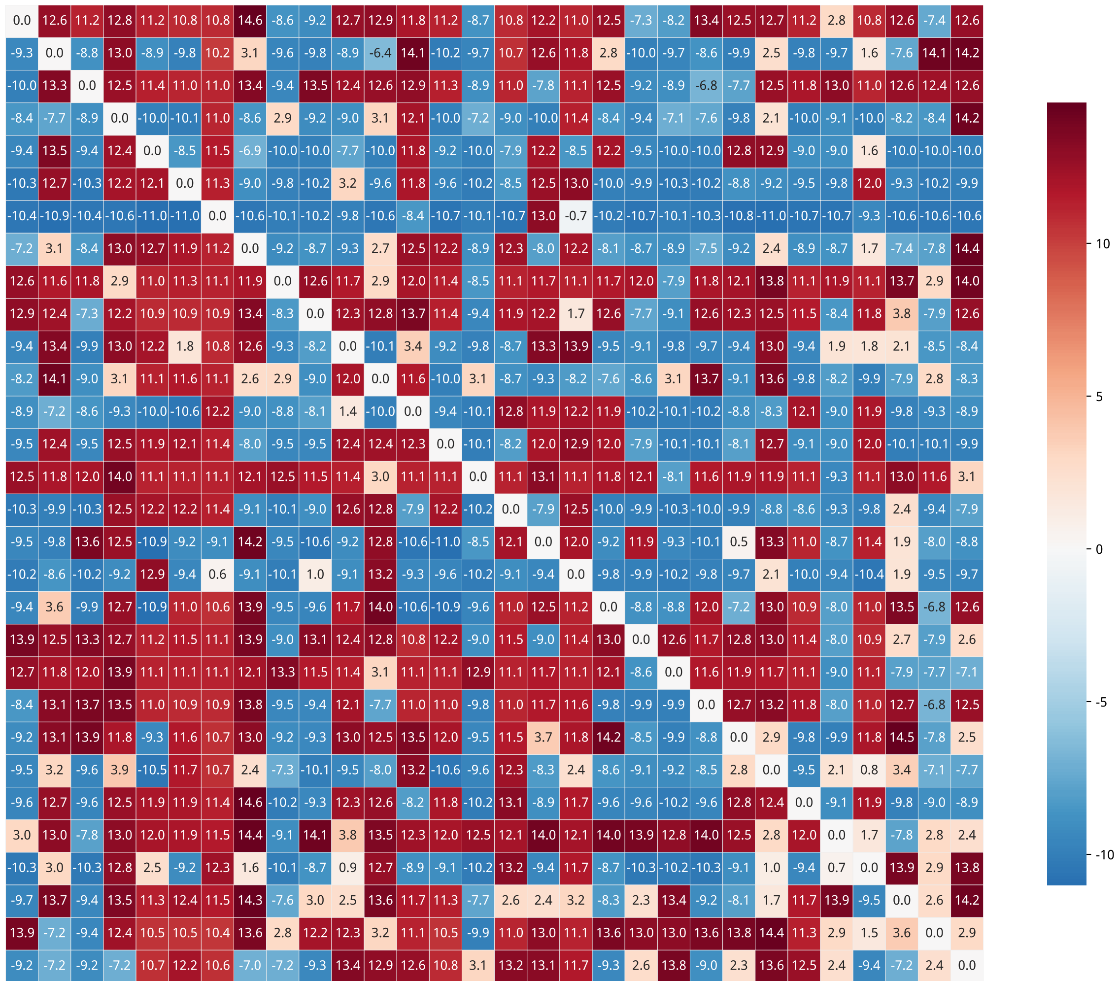
对手策略 \psi^{-1}
