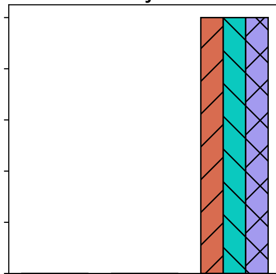
rojo
