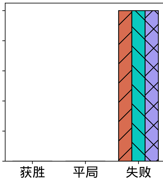
randomBiasedAI
