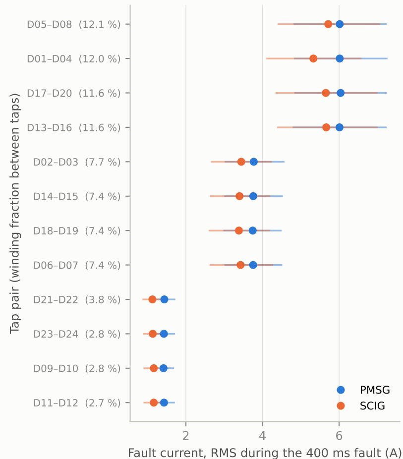
Inter-turn short-circuits
