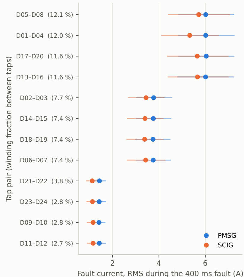
Inter-turn short-circuits
