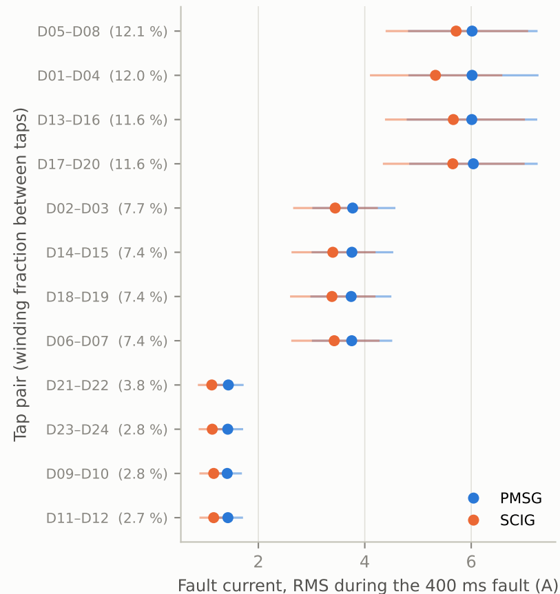
Inter-turn short-circuits
