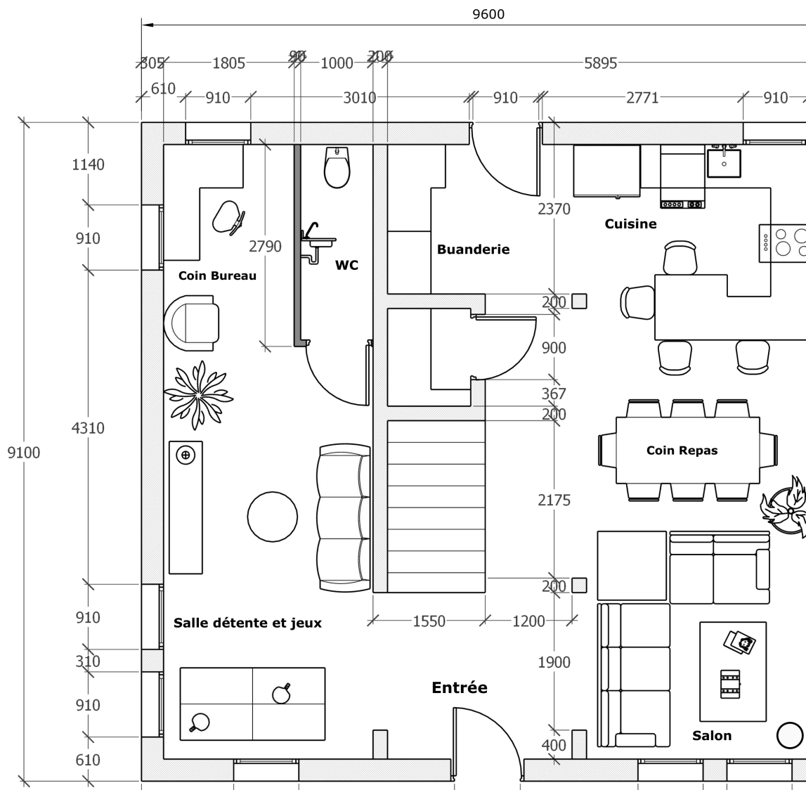
Plan de sol fourni (cotes réelles).
