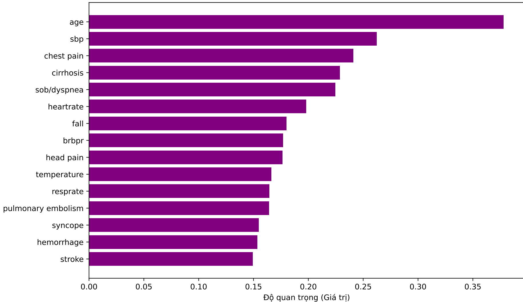
Top 15 Đặc trưng Quan trọng Toàn cục - LogisticRegression
