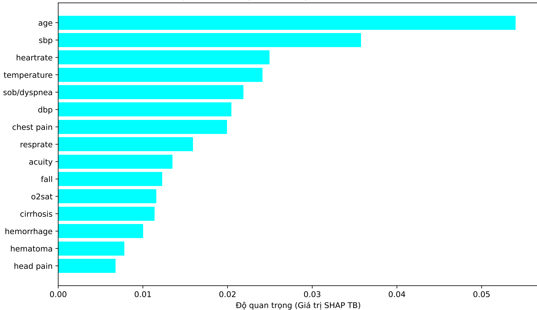
Top 15 Đặc trưng Quan trọng Toàn cục - MLPClassifier
