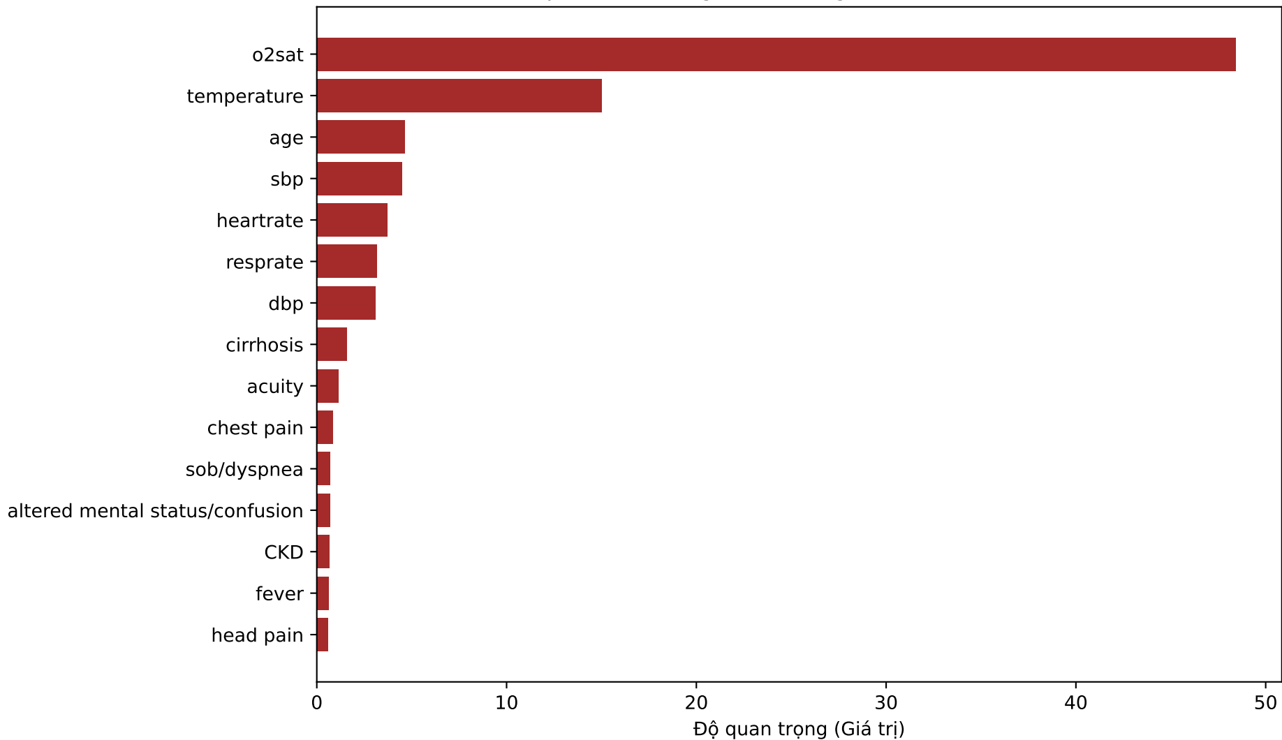
Top 15 Đặc trưng Quan trọng Toàn cục - CatBoost
