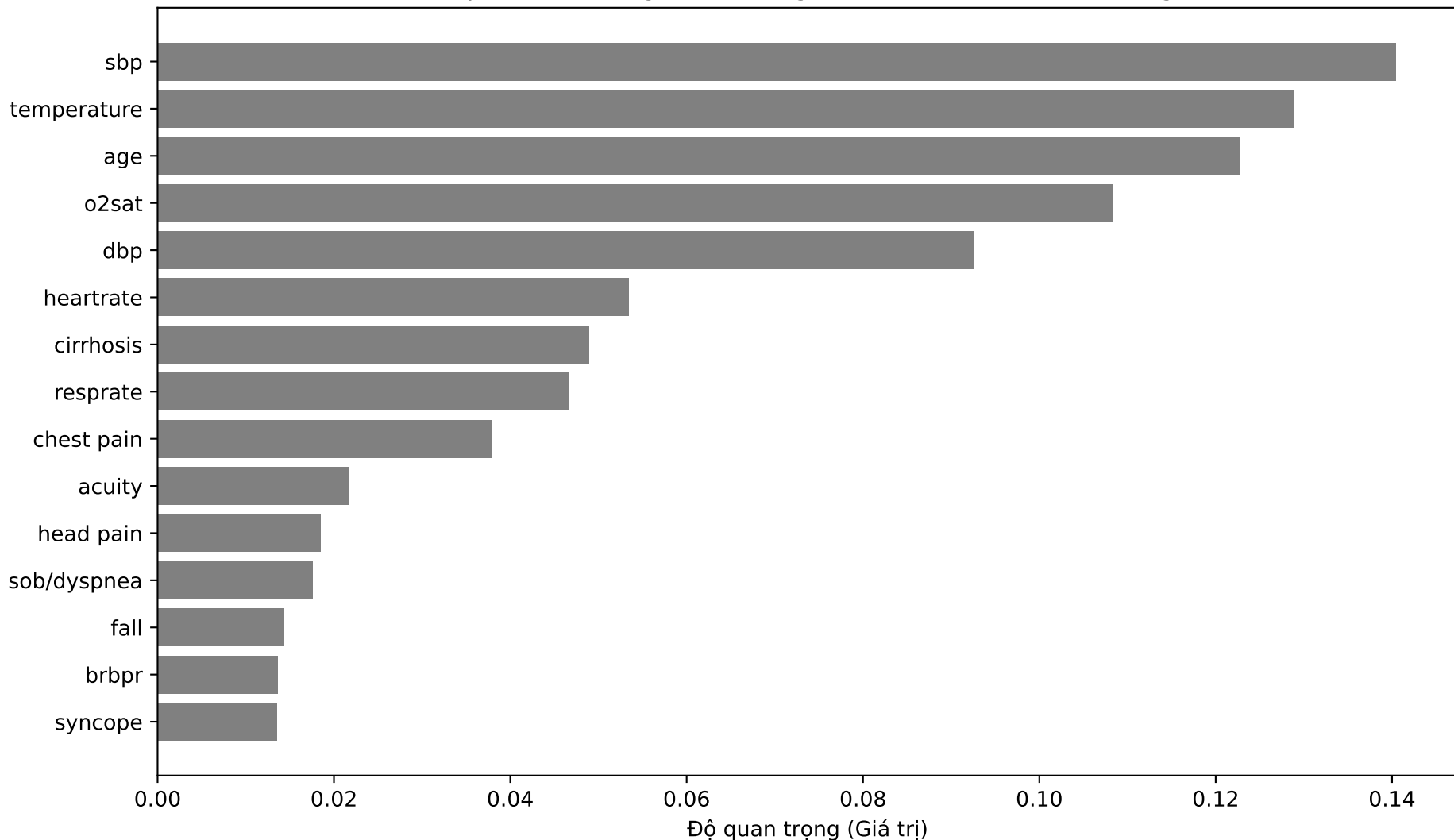
Top 15 Đặc trưng Quan trọng Toàn cục - GradientBoosting
