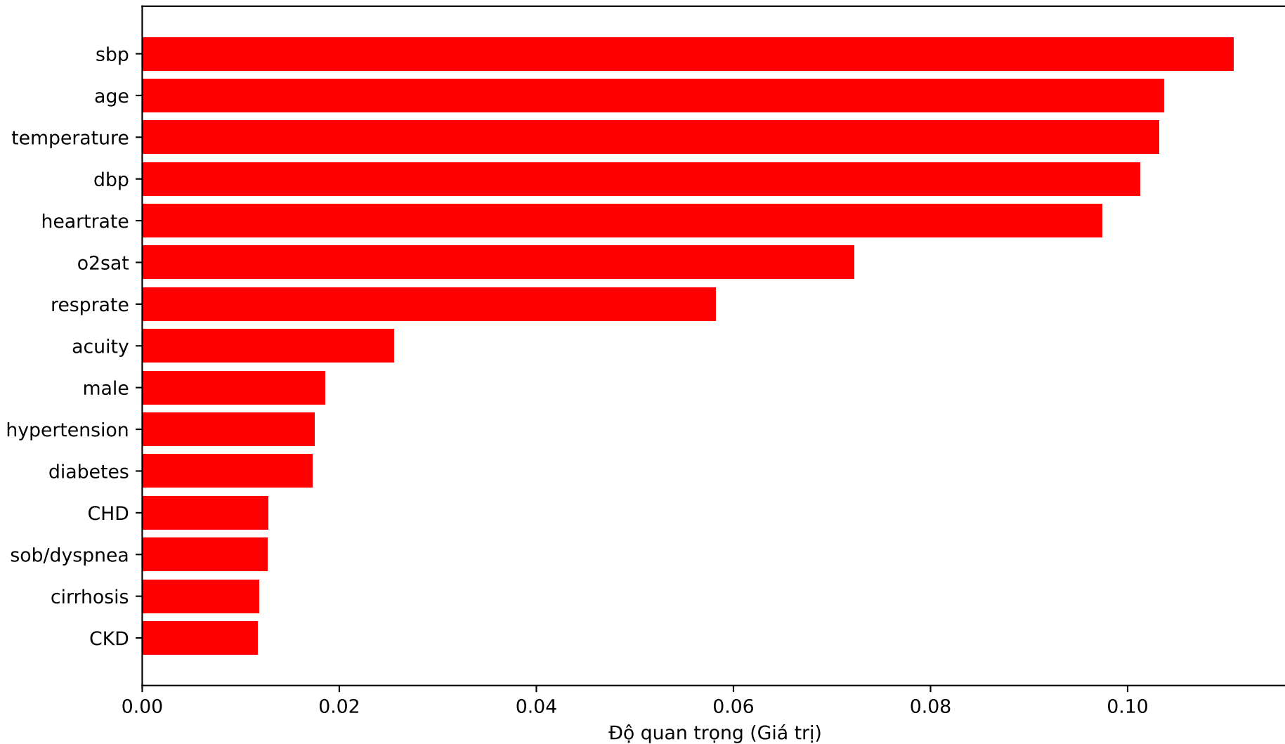
Top 15 Đặc trưng Quan trọng Toàn cục - RandomForest
