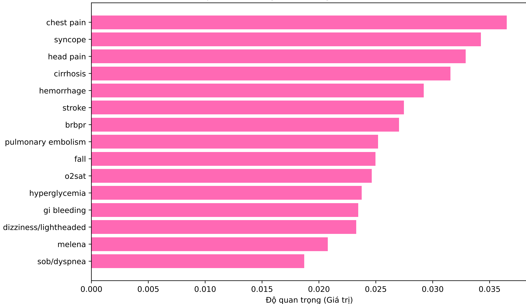
Top 15 Đặc trưng Quan trọng Toàn cục - XGBoost
