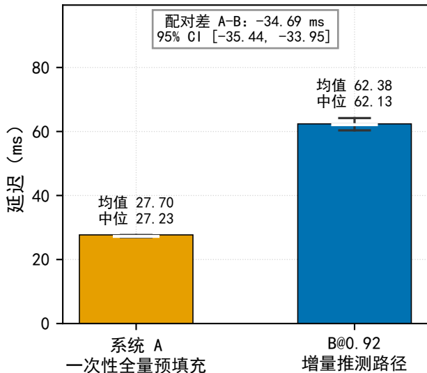
(a) 最后段到达→候选选择/计算就绪
