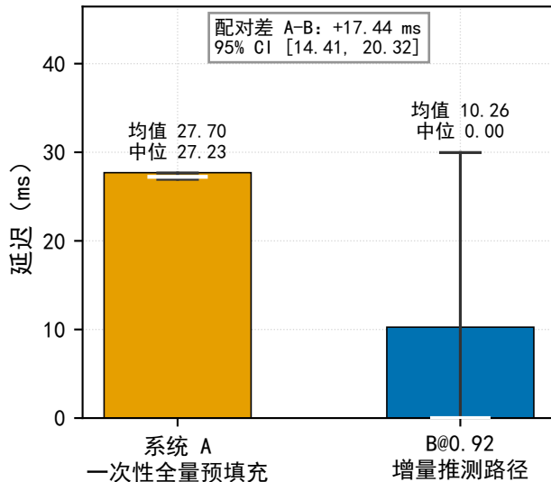
(b) oracle TTFT eff : 时延乐观下界
