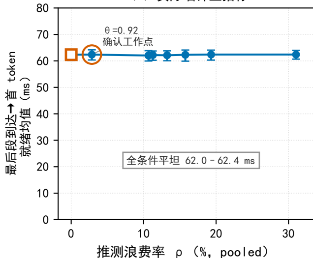
(b) 实际墙钟主指标
