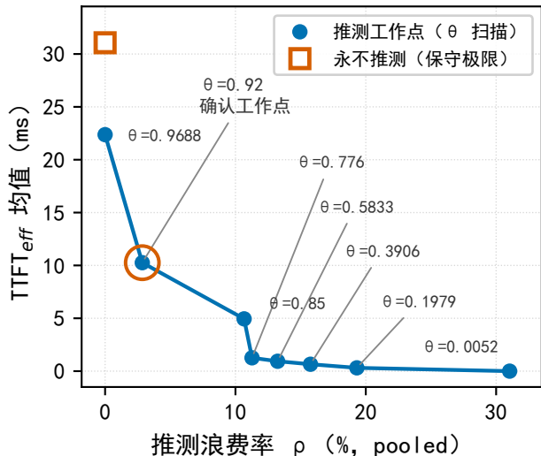
(a) oracle 口径: \text{TTFT}_{\text{eff}} 时延乐观下界
