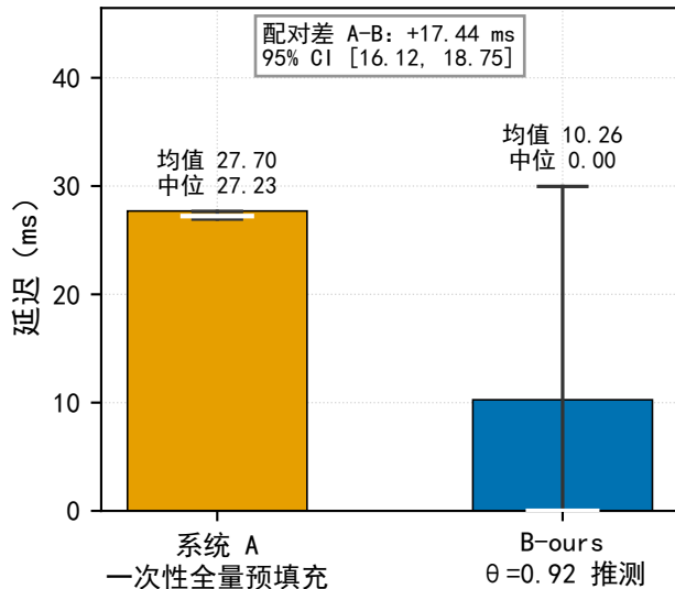
(b) oracle \text{TTFT}_{\text{eff}} : 时延乐观下界
