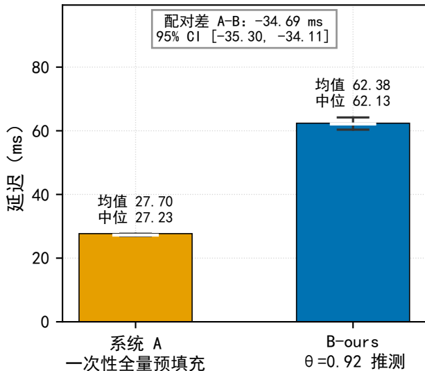
(a) 实际墙钟：最后段到达→首 token 就绪
